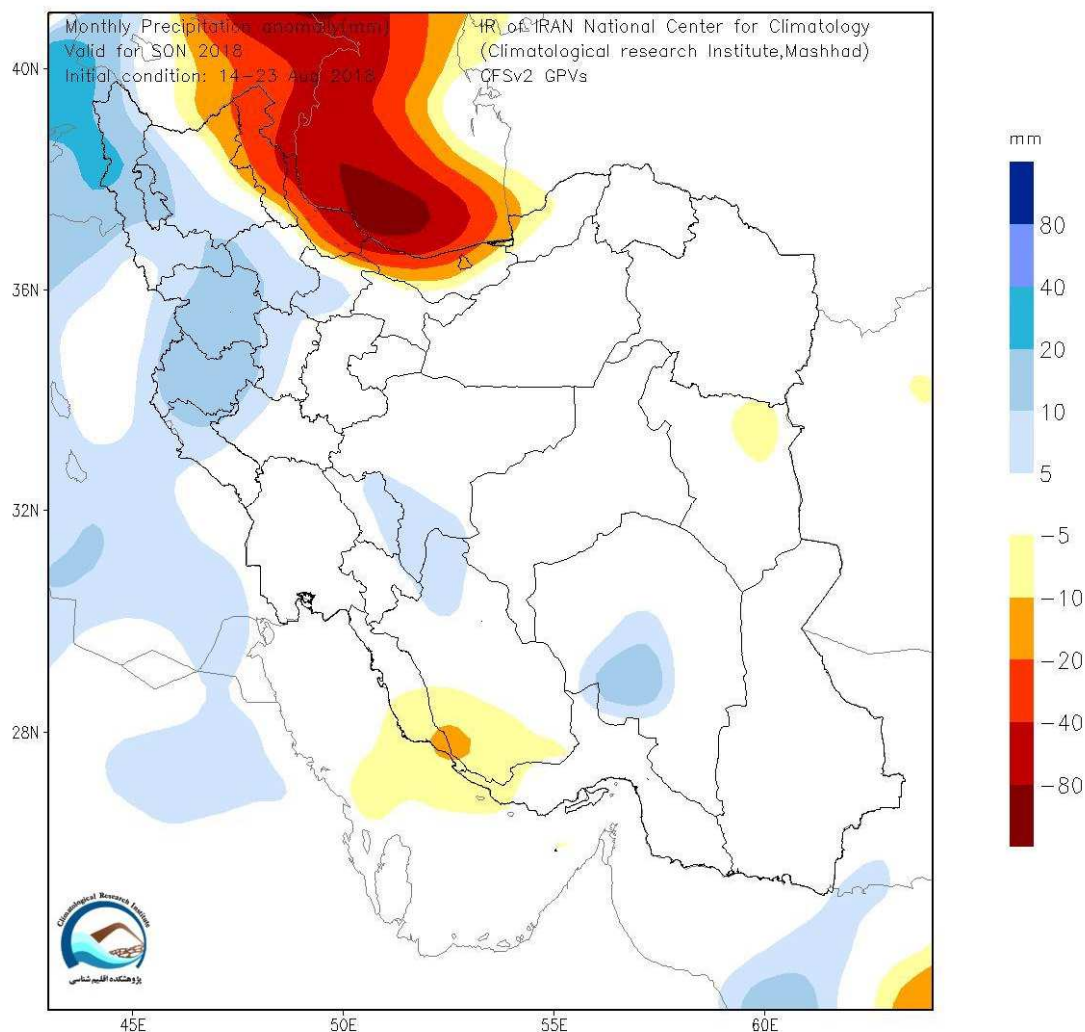
نقشه ۹- پیش بینی بارش شهریور تا آبان ۹۷
