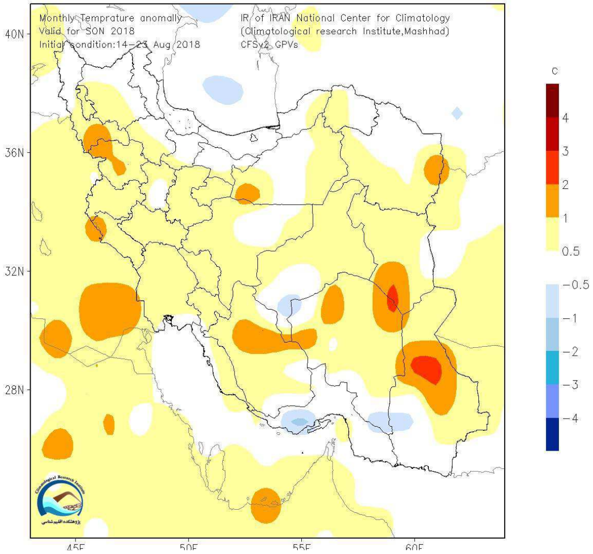
نقشه ۱۰- پیش بینی میانگین دمای شهریور تا آبان ۹۷
